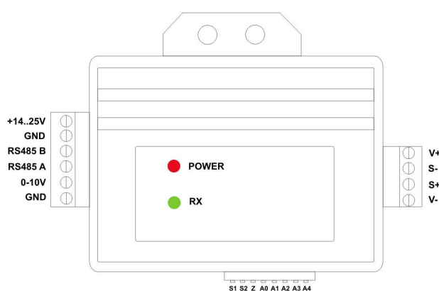
Rys. 1 Opis złączy
