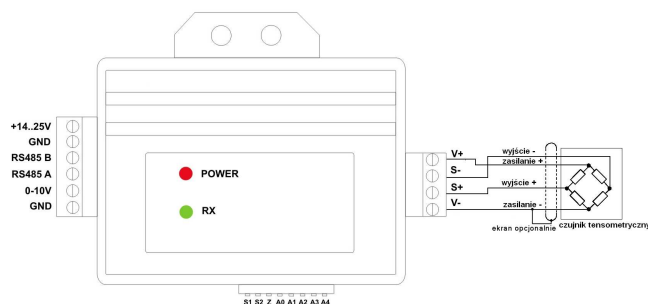
Rys. 2 Podłączenie czujnika do urządzenia
