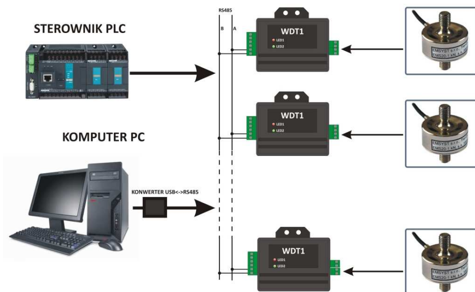
Rys. 3 Połączenie na magistrali MODBUS
