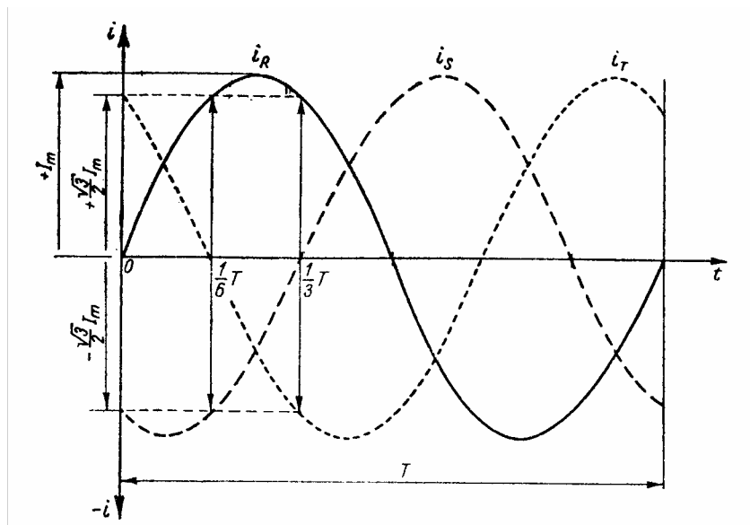
Rys.3. Przebiegi prądów w trzech fazach uzwojenia stojana
