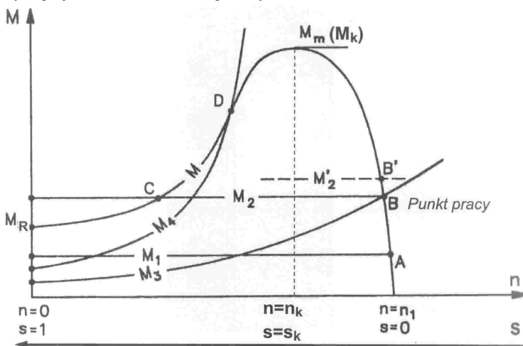
Rys. 6. Naturalna charakterystyka mechaniczna silnika asynchronicznego
