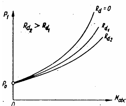
Rys. 18. Charakterystyki mocy pobieranej z sieci przez silnik pierścieniowy w funkcji obciążenia
