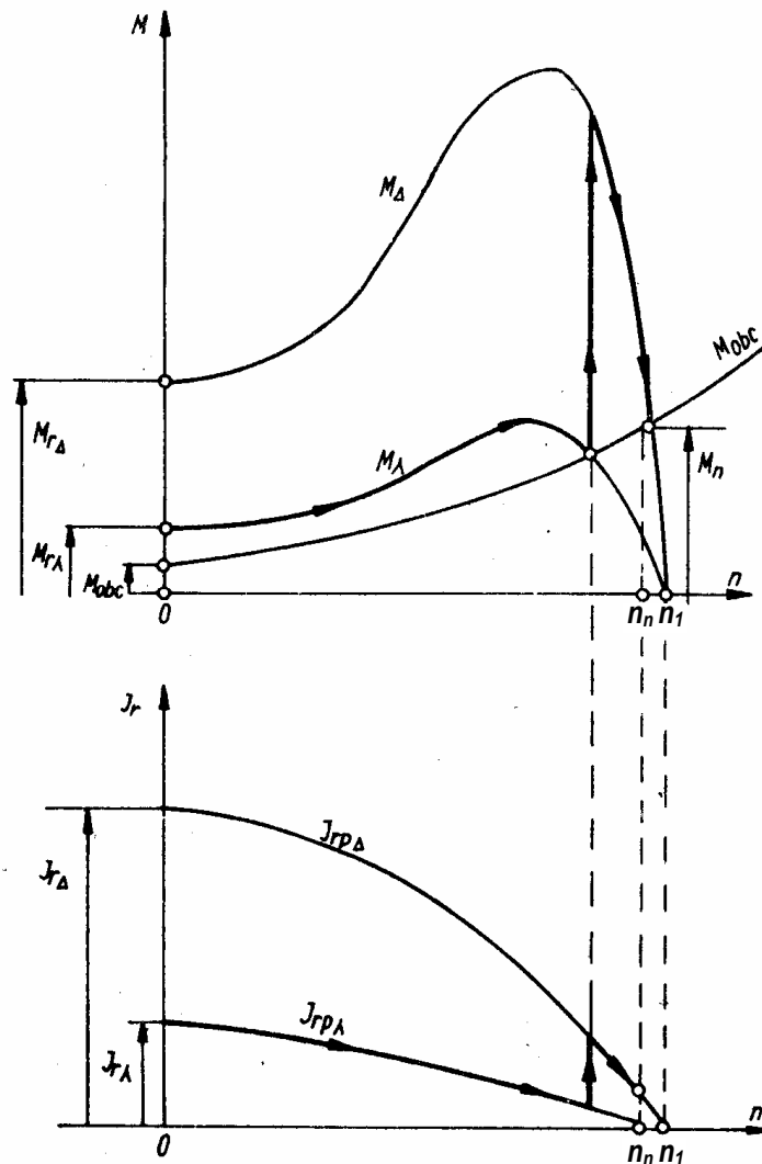
Rys.8. Przebieg momentu oraz prądów przy rozruchu silnika klatkowego z przełącznikiem gwiazda-trójkąt
