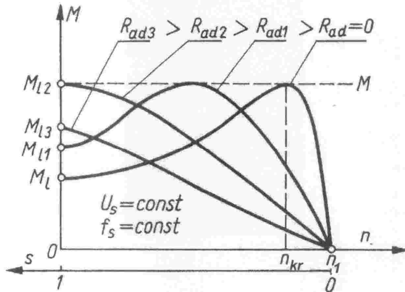
Rys.13. Charakterystyki mechaniczne silnika pierścieniowego przy różny rezystancjach w obwodzie wirnika
