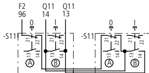
Dwa łączniki dwuprzyciskowe
