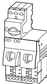
MSC-D Rozrusznik bezpośredni
