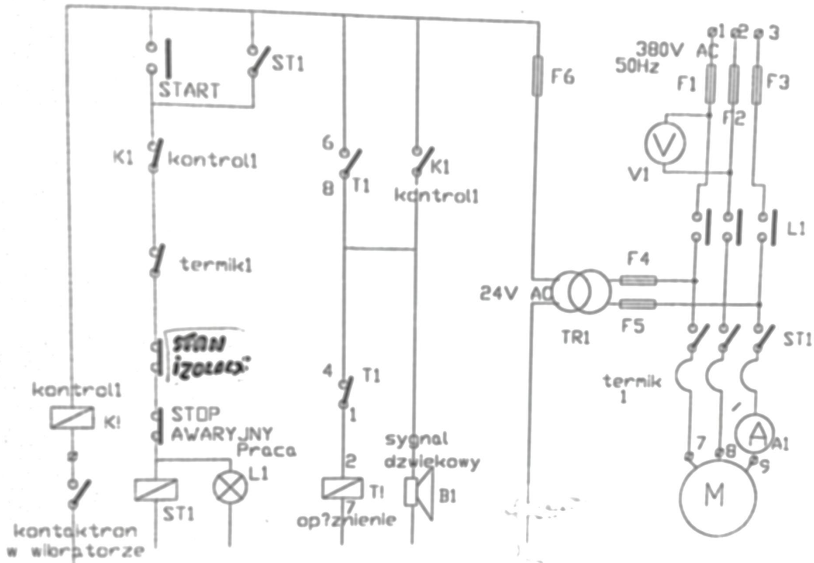
Połączenia w sterowniku wibrosondy VKG
