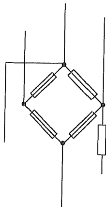
Sonda lettura pressione tipo strangaugé
