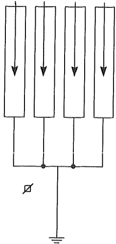
Scaricatore extratensioni
